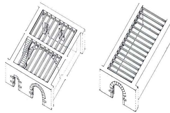
Figura 3.- Esquemes comparatius de les dues tipologies comentades: a l'esquerra, amb arc central o travesser, i a la dreta, la tradicional.
