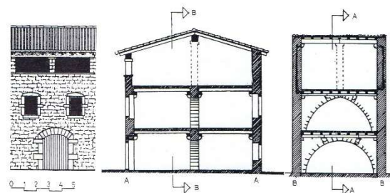
Figura 4.- Esquema d'alçat i seccions típic d'una casa medieval de Banyoles, amb arcs travessers.
